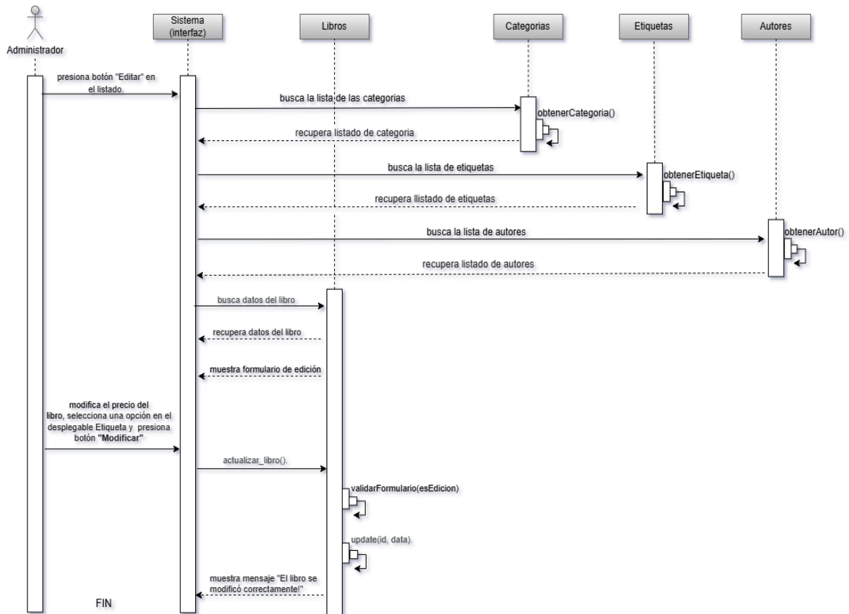
Fig. 2.10.2.2.1 Secuencia Gestionar catálogo (editar un libro).
