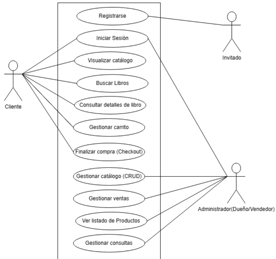
Fig. 2.9.1 Diagrama de Casos de Usos
