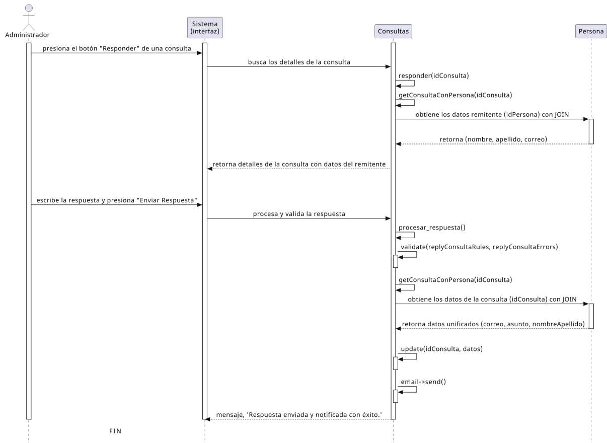
Fig. 2.10.6.2 Secuencia Gestionar Consultas
