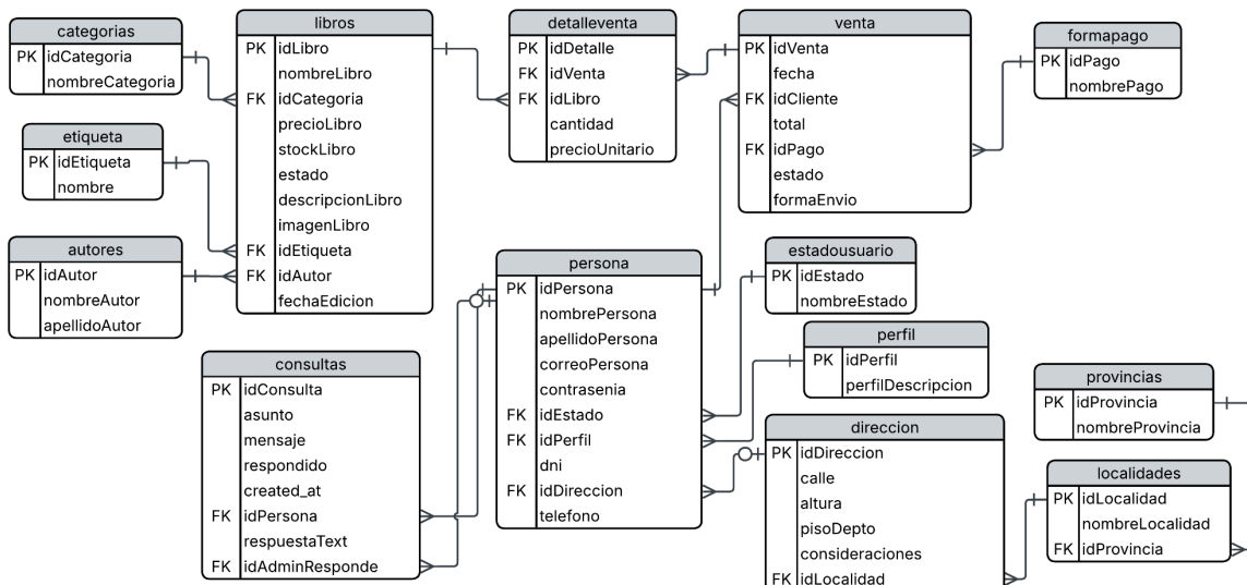
Fig. 2.11.1 Diagrama de Modelo de datos
